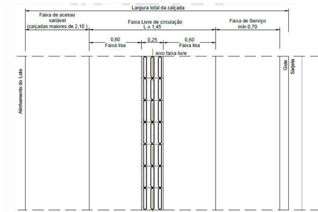
Figura 61 – Sinalização tátil no eixo da faixa livre de circulação com largura \geq 1,45 m
